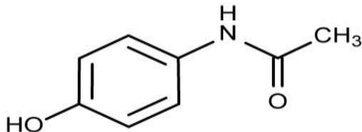
Gambar 2. Struktur Parasetamol
