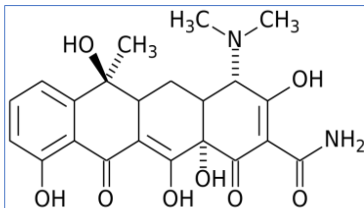
Gambar 1. Struktur Tetrasiklin
