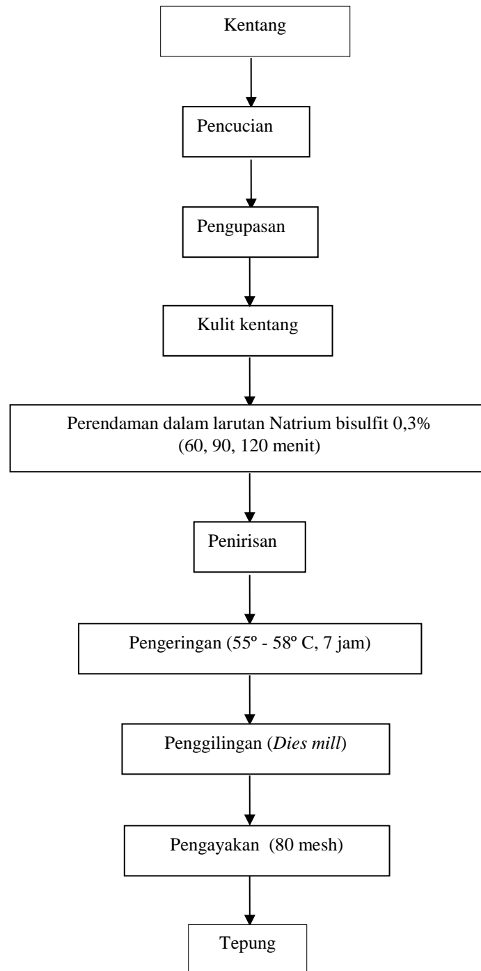
Gambar 1. Proses Pembuatan tepung Kulit Kentang
